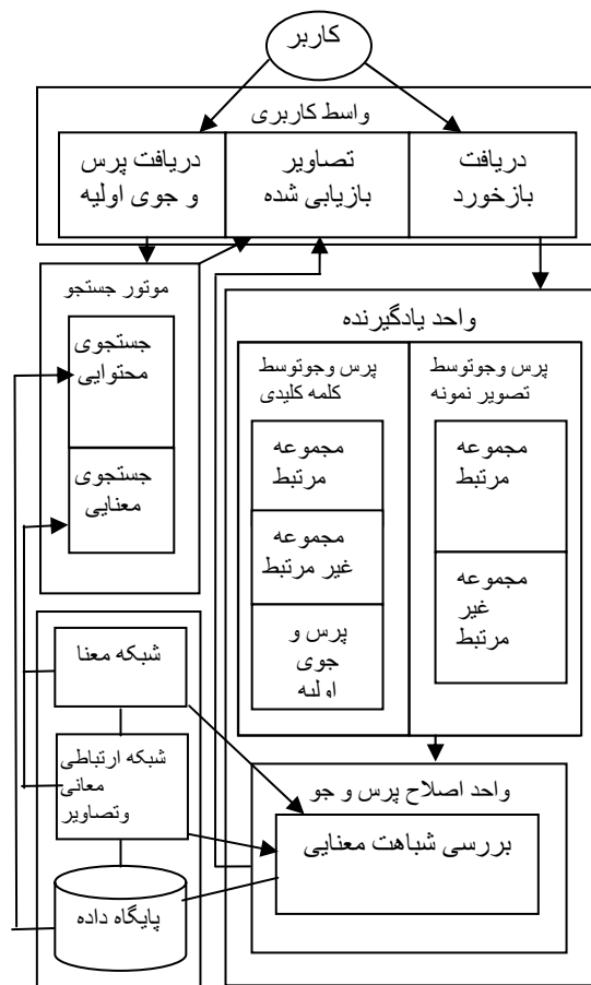
شکل ۱. مؤلفه های اصلی سیستم پیشنهادی
