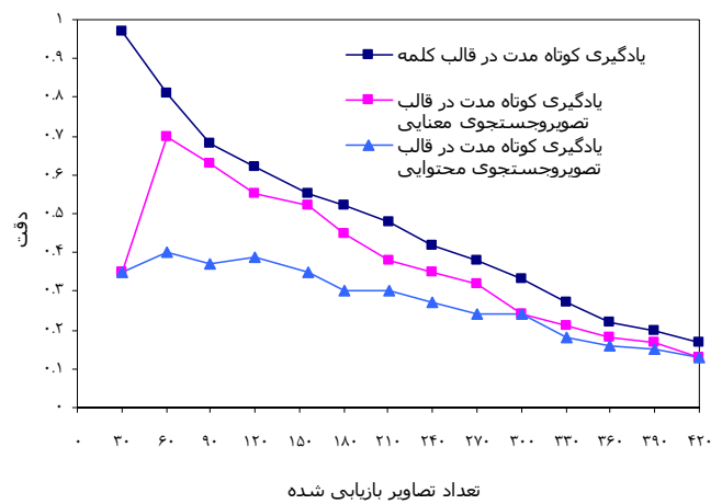
شکل ۷. نمودار دقت سیستم پیشنهادی
